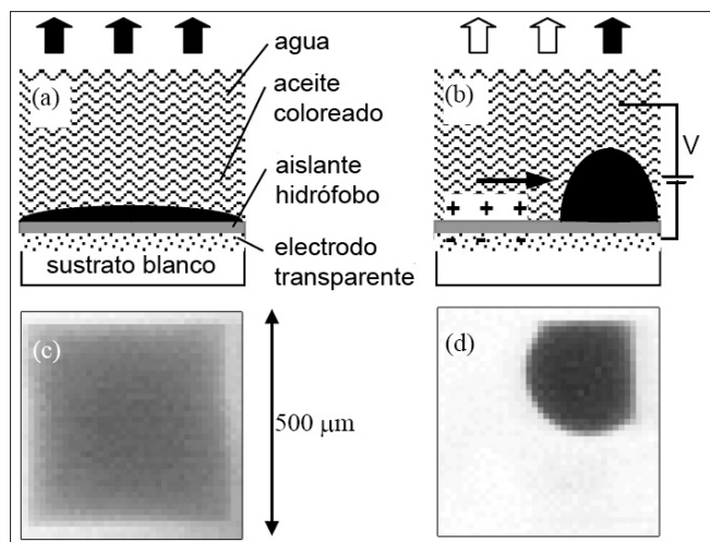
Figura 4. Principio de funcionamiento de la pantalla de electrohumedecimiento. Esquema en sección: (a) sin aplicar tensión presenta una película homogénea de aceite; (b) aplicando corriente continua se causa una contracción del aceite. Las fotografías en vista superior (c) y (d) muestran como el aceite se retrae ante un electrodo.
