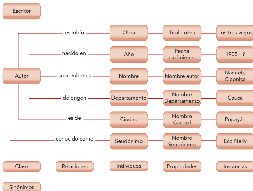
Figura 3. Ejemplificación de una ontología basada en un tesoro
