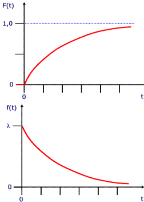
FIGURA 5 – Modelo de Distribución Exponencial
