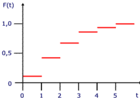
FIGURA 3 – Modelo de Distribución Binomial
