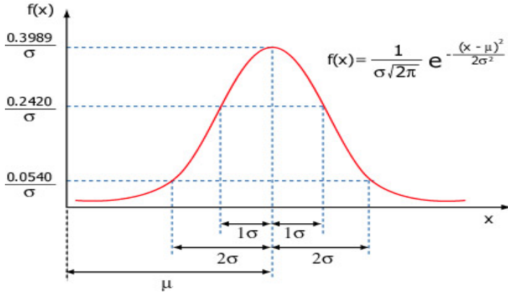
FIGURA 4 – Función de densidad de probabilidad normal
